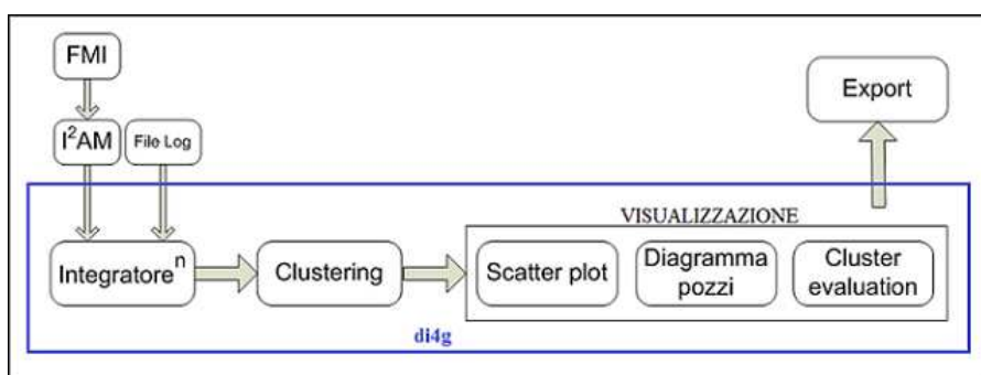
Fig. 1. Workflow di di4g
