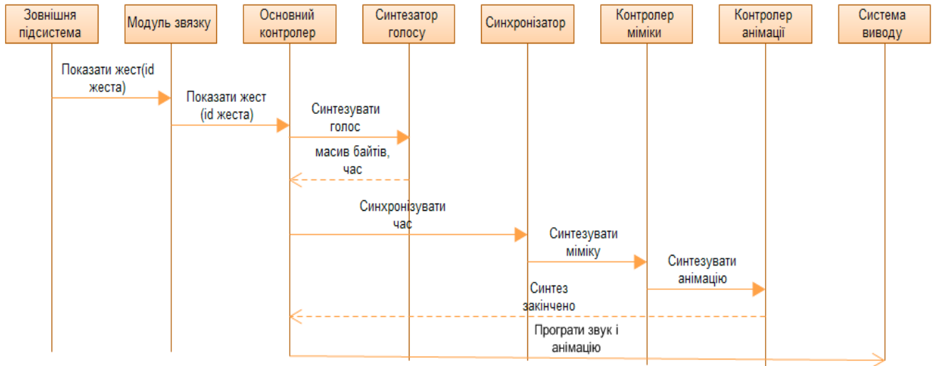
Рис. 5. Діаграма послідовностей
