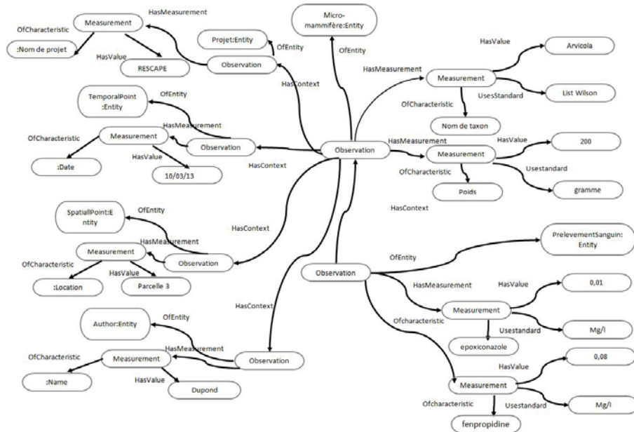
Figure 4 : Exemple d'instanciation dans OBOE
