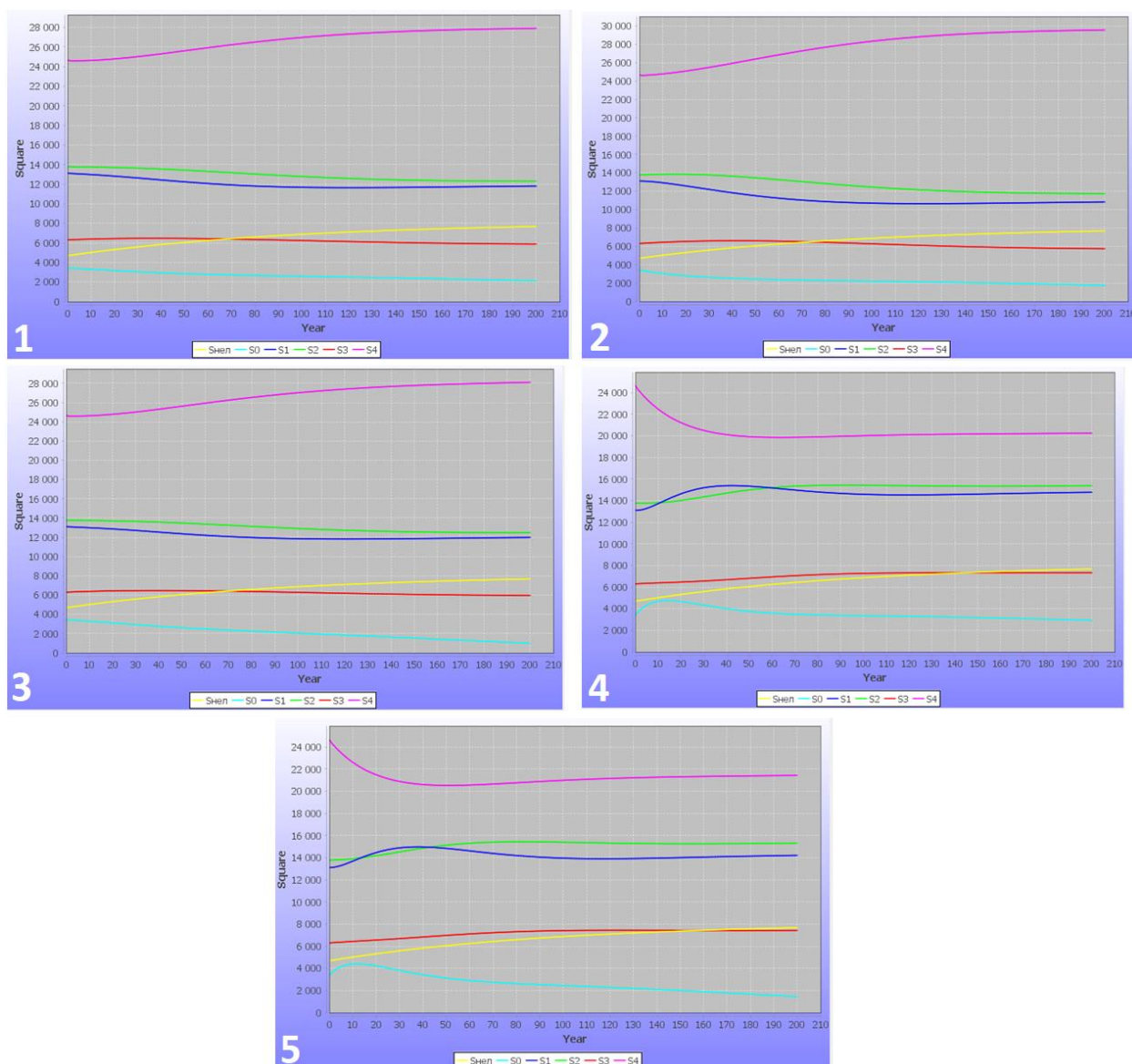
Рис. 2. Графики динамики лесных ресурсов по 5 сценариям
